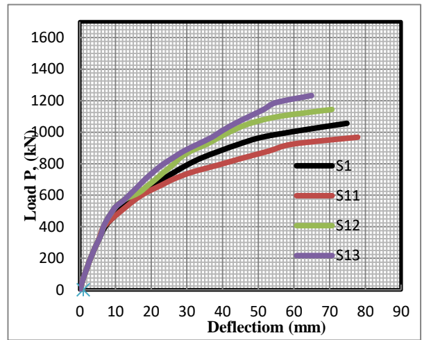
(d) Effect of shear studs diameter ( D_b )
